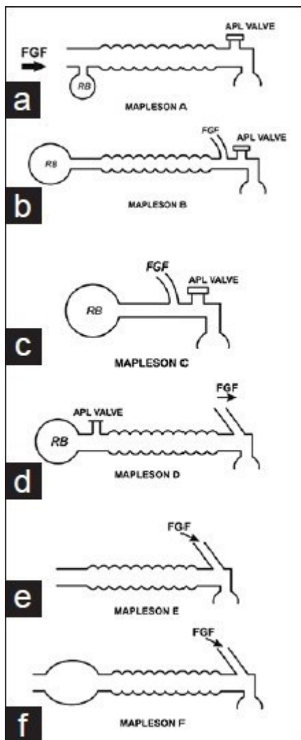
Slika 8. Maplesonovi linearni dihalni sistemi a-f (12).
