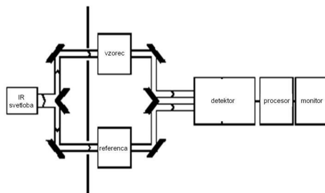
Slika 14. Shema merjenja koncentracije ogljikovega dioksida s pomočjo infrardeče absorpcijske spektrografije.
