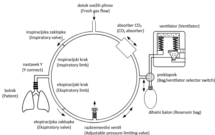
Slika 7. Krožni dihalni sistem in njegovi sestavni deli (J).
