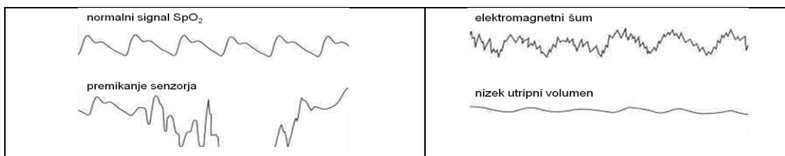
Slika 12. Oblika signala pulznega oksimetra (4).
