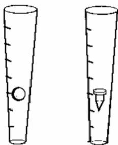
Slika 4. Pretočni merilnik s krogličnim in valjnim plavcem.
