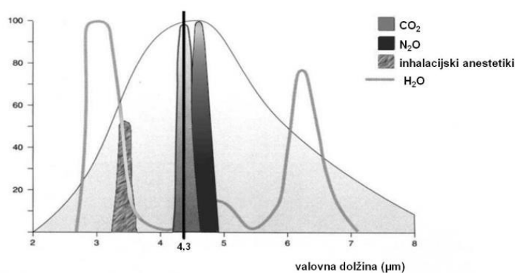
Slika 15. Spekter infrardeče svetlobe, ki jo absorbirajo ogljikov dioksid in anestezijski plini.
