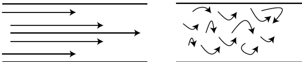
Slika 10: Laminarni (levo) in vrtinčast (desno) tok tekočine.
