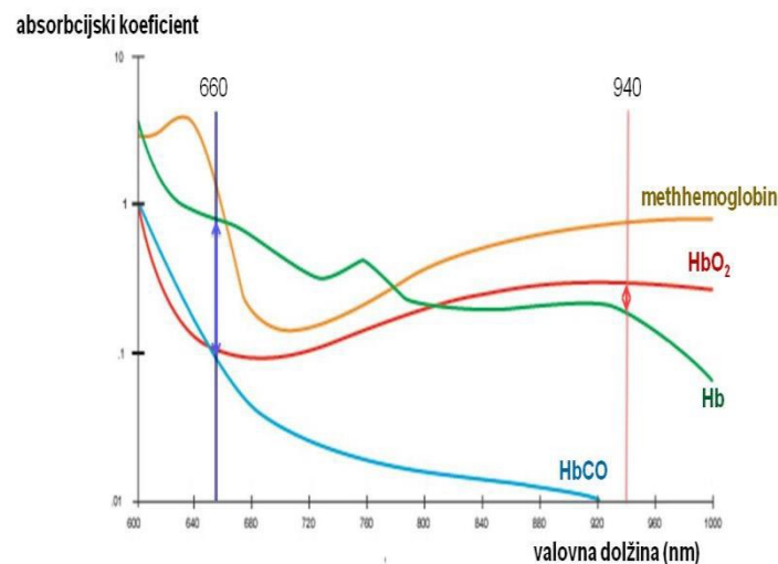
Slika 10. Absorpcijski spekter elektromagnetnega valovanja za različne oblike hemoglobina
