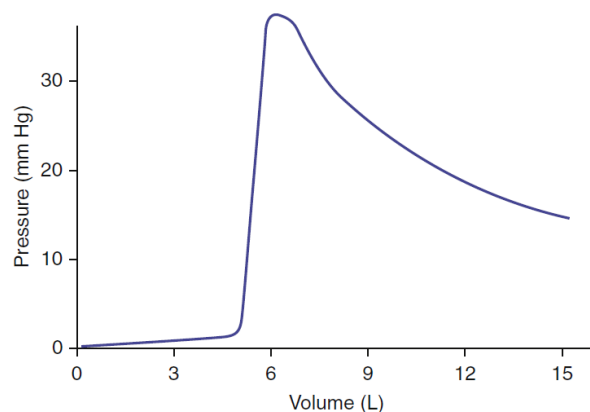
Slika 8: Varovalna funkcija anestzijskega dihalnega balona (levo) in dinamična sprememba tlaka v balonu med njegovim polnjenjem.
