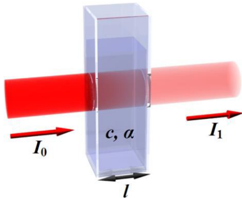
Slika 9. Beer-Lambertov zakon
